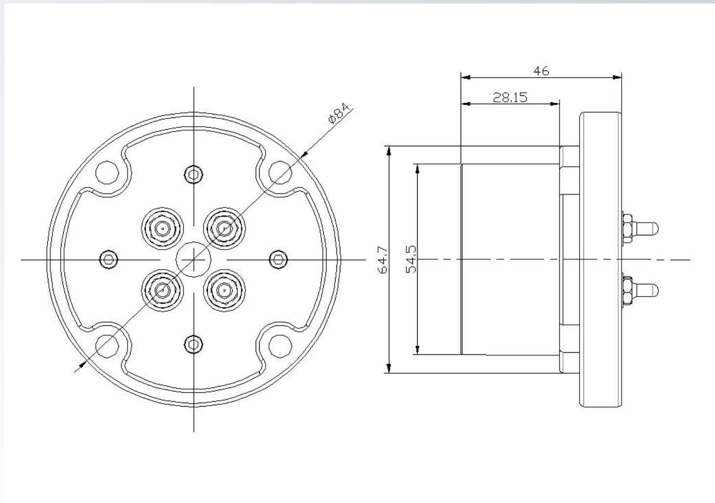
尺寸图
